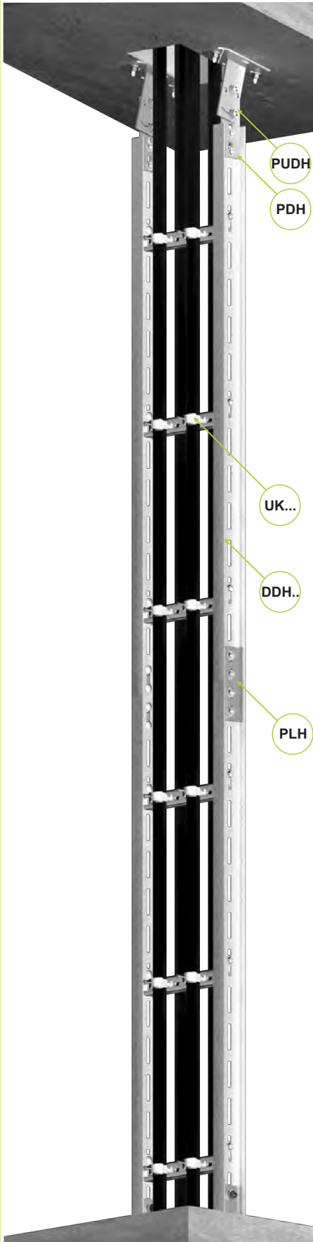
Пример монтажа кабельроста DDH (крепление кабельроста к стене)
