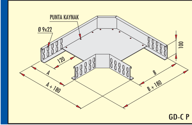
Ağır Hizmet 90° Dönüş Elemanı h=100 mm PASLANMAZ SAC (Cr-Ni) 90° Heavy Duty Flat Bend h=100 mm Stainless Steel (Cr-Ni) Сверхмощные угловые элементы 90°
