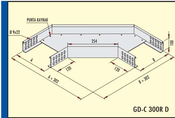
Ağır Hizmet 90° Dönüş Elemanı 300 Radüs (h=100 mm) 90° Heavy Duty Flat Bend Radius 300 (h=100 mm) Сверхмощные угловые элементы 90° (Радиус 300)
