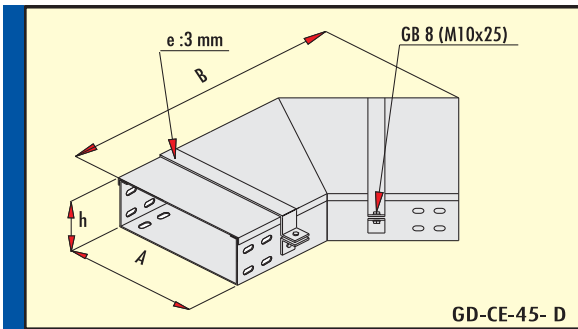
135° Dönüş Elemanı 135° Flat Bend Element 135° Квартир Стибают Элемент
