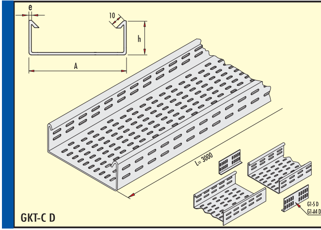
Ğir Hizmet Tipi Kablo Kanalı (h=100 mm) Heavy Duty Cable Tray (h=100 mm) Сверхмощные кабельные лотки
