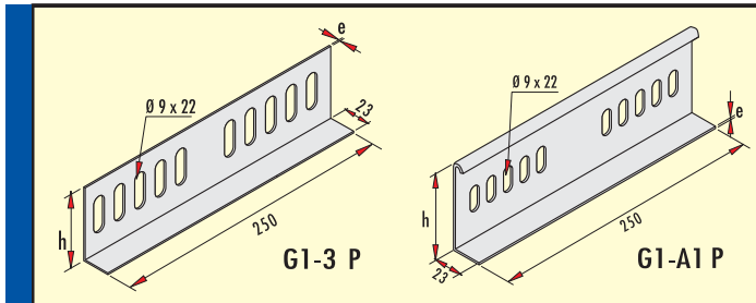
Ek Parçası h=50 mm PASLANMAZ SAC (Cr-Ni) Jointing Piece h=50 mm Stainless Steel (Cr-Ni)
