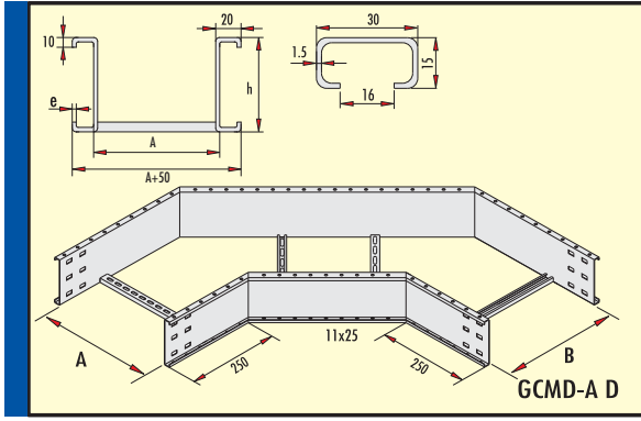
90° Dönüş Elemanı 300 Radius (h=150 mm) 90° Flat Bend Element Radius 300 (h=150 mm) 90° Квартир Стибают Элемент
