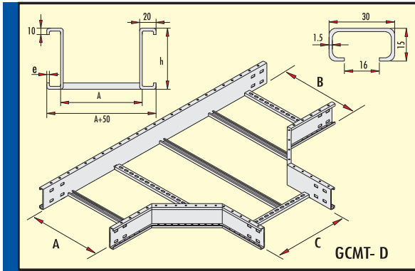
"T" Bağlantı Elemanı 300 Radius (h=100 mm) Tee "T" Element Radius 300 (h=100 mm) Мишень "Т" Квартира Стибают Элемент
