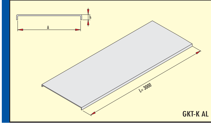
Kablo Kanal Kapağı (5052 ALÜMİNYUM ALAŞIM) Cover For Cable Tray (5052 Aluminium Alloy) Крышки для кабельных лотков
