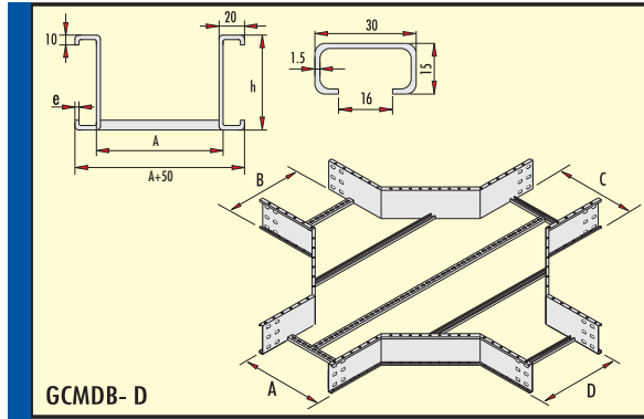
Dörtlü Bağlantı Elemanı 300 Radüs (h=100 mm) Crossing Element Radius 300 (h=100 mm) Пересечение Элемента
