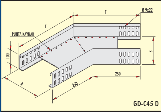
135° Ağır Hizmet Dönüş Elemanı (h=100 mm) 135° Heavy Duyt Flat Bend (h=100 mm) Плоский Изгиб 135°
