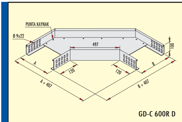
Ağır Hizmet 90° Dönüş Elemanı 600 Radüs (h=100 mm) 90° Heavy Duty Flat Bend Radius 600 (h=100 mm) Сверхмощные угловые элементы 90° (Радиус 600)
