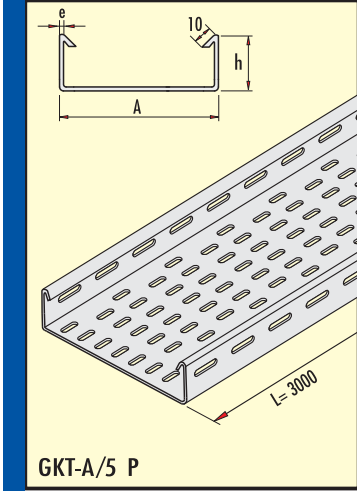
Ağır Hizmet Tipi Kablo Kanalı h=50 mm PASLANMAZ SAC (Cr-Ni) Heavy Duty Cable Tray h=50 mm Stainless Steel (Cr-Ni) Сверхмощные кабельные лотки
