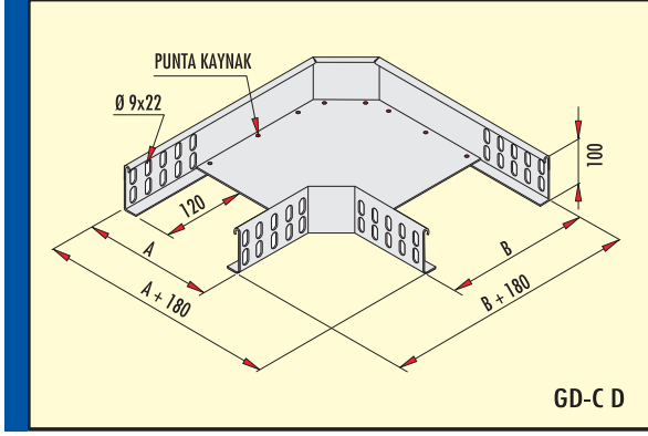
Ağır Hizmet 90° Dönüş Elemanı (h=100 mm) 90° Heavy Duty Flat Bend (h=100 mm) Сверхмощные угловые элементы 90°
