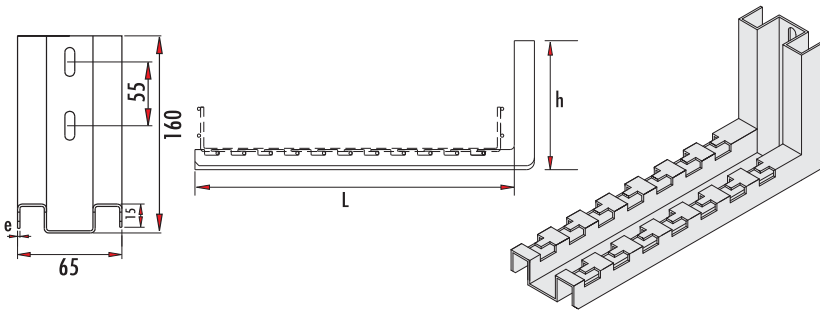
Tel Kanal Konsolu Wire-mesh bracket Проволочная консоль
