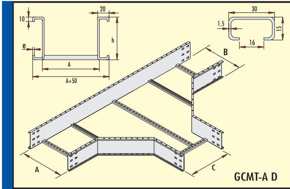
"T" Dönüş Elemanı 300 Radius (h=150 mm) Tee "T" Flat Bend Element Radius 300 (h=150 mm) Мишень "Т" Квартира Стибают Элемент
