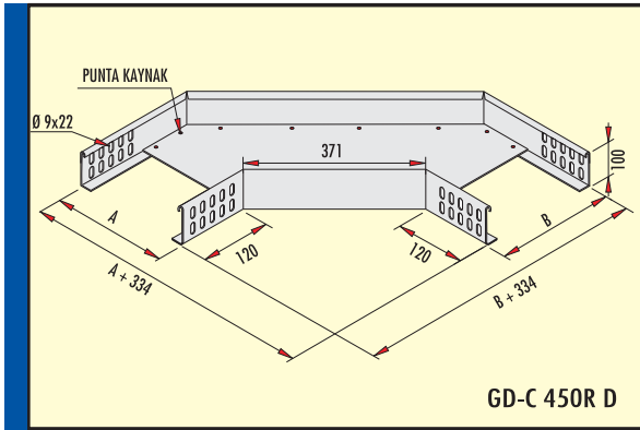
Ağır Hizmet 90° Dönüş Elemanı 450 Radüs (h=100 mm) 90° Heavy Duty Flat Bend Radius 450 (h=100 mm) Сверхмощные угловые элементы 90° Радиус 450
