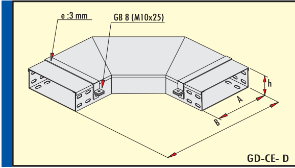
90° Dönüş Elemanı 300 Radius (h=100 mm) 90° Flat Bend Element Radius 300 (h=100 mm) 90° Квартир Стибают Элемент
