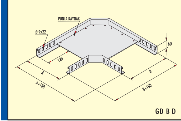
Ağır Hizmet 90° Dönüş Elemanı (h=60 mm) 90° Heavy Duty Flat Bend (h=60 mm) Сверхмощные угловые элементы 90°
