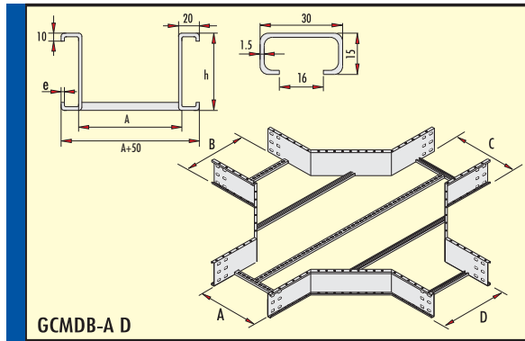
Dörtlü Bağlantı Elemanı 300 Radüs (h=150 mm) Crossing Element Radius 300 (h=150 mm) Пересечение Элемента
