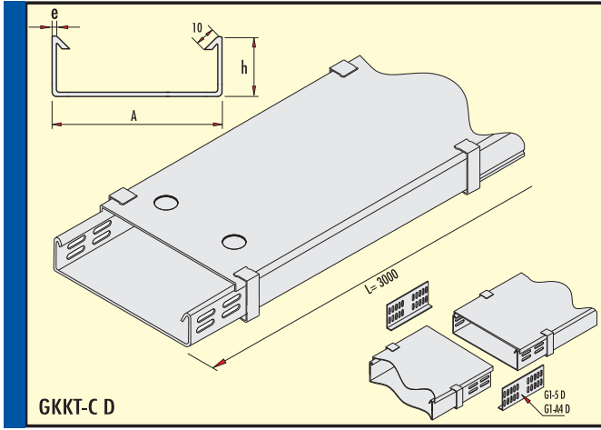
Deliksiz Ğir Hizmet Tipi Kablo Kanalı (h=100 mm) Non Perforated Heavy Duty Cable Trays With Cover (h=100 mm) Сверхмощные кабельные лотки с крышкой
