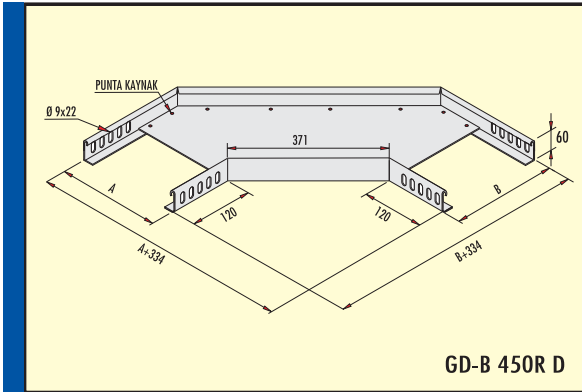
Ağır Hizmet 90° Dönüş Elemanı 450 Radyüs (h=60 mm) 90° Heavy Duty Flat Bend Radius 450 (h=60 mm) Сверхмощные угловые элементы 90° Радиус 450
