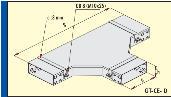
"T" Bağlantı Elemanı 300 Radius (h=100 mm) Tee "T" Element Radius 300 (h=100 mm) Мишень "Т" Квартира Стибают Элемент
