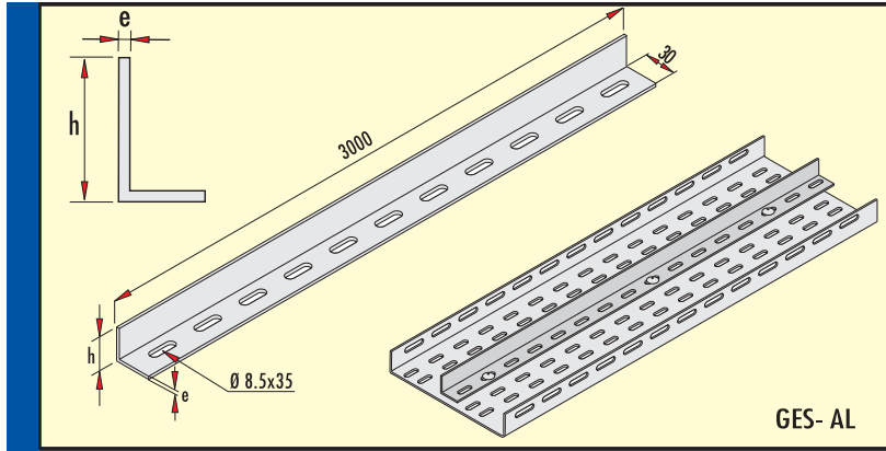
Seperator (5052 ALÜMİNYUM ALAŞIM) Separator (5052 Aluminium Alloy) Сепаратор
