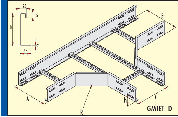
"T" Bağlantı Elemanı 300 Radius (h=100 mm) Tee "T" Element Radius 300 (h=100 mm) Мишень "Т" Квартира Сгибает Элемент
