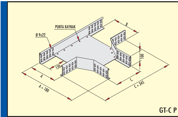
Ağır Hizmet T Bağlantı Elemanı h=100 mm PASLANMAZ SAC (Cr-Ni) Heavy Duty Tees "T" h=100 mm Stainless Steel (Cr-Ni) Сверхмощные «Т» образные соединительные элементы
