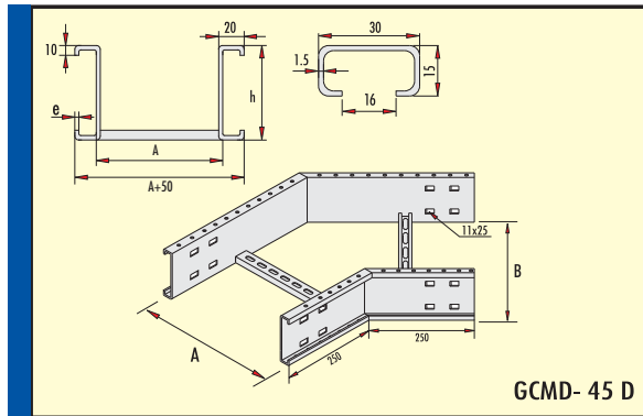
135° Dönüş Elemanı (h=100 mm) 135° Flat Bend Element (h=100 mm) 135° Квартир Стибают Элемент
