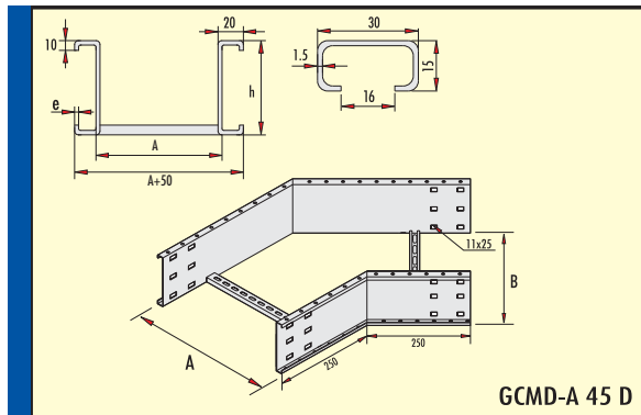
135° Dönüş Elemanı (h=150 mm) 135° Flat Bend Element (h=150 mm) 135° Квартир Стибают Элемент
