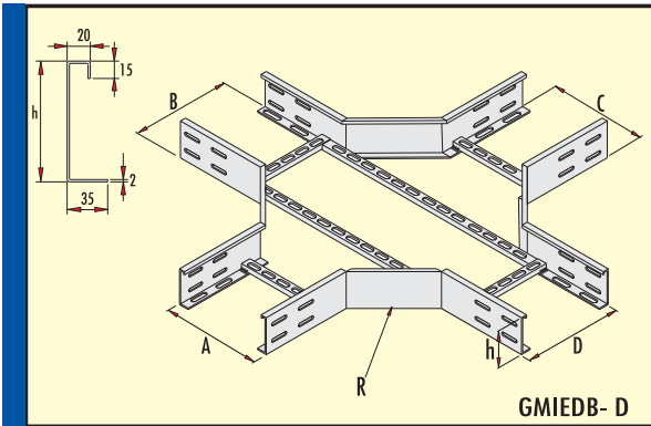
Dörtlü Bağlantı Elemanı 300 Radius (h=100 mm) Crossing Element Radius 300 (h=100 mm) Пересечение Элемента
