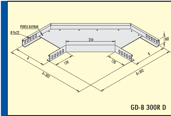
Ağır Hizmet 90° Dönüş Elemanı 300 Radyüs (h=60 mm) 90° Heavy Duty Flat Bend Radius 300 (h=60 mm) Сверхмощные угловые элементы 90° (Радиус 300)
