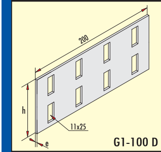
Ek Parçası Jointing Piece
