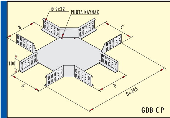
Ağır Hizmet Dörtlü Bağlantı Elemanı h=100 mm PASLANMAZ SAC (Cr-Ni) Heavy Duty Crossing h=100 mm Stainless Steel (Cr-Ni) Сверхмощные крестообразные соединительные элементы
