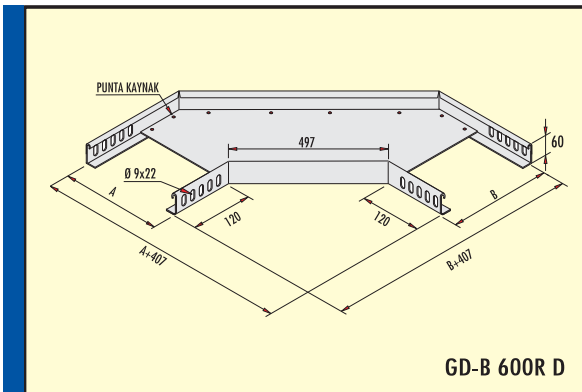
Ağır Hizmet 90° Dönüş Elemanı 600 Radyüs (h=60 mm) 90° Heavy Duty Flat Bend Radius 600 (h=60 mm) Сверхмощные угловые элементы 90° (Радиус 600)
