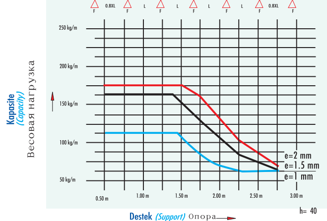
Eşit aralıklarla destekleyiniz (Equal distance Support) Устанавливать на равных промежутках
