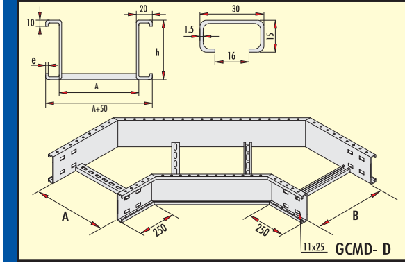
90° Dönüş Elemanı 300 Radius (h=100 mm) 90° Flat Bend Element Radius 300 (h=100 mm) 90° Квартир Стибают Элемент
