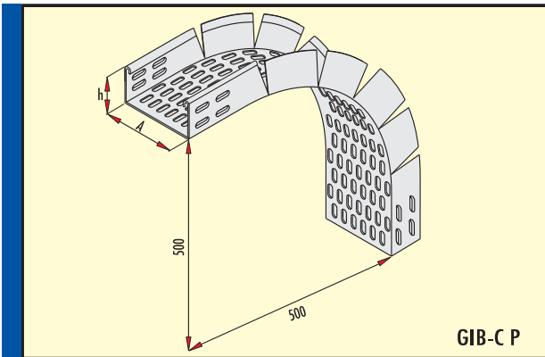
Ağır Hizmet İç-Dış Bükü Elemanı h=100 mm PASLANMAZ SAC (Cr-Ni) Heavy Duty Inside and Outside Vertical Bend h=100 mm Stainless Steel (Cr-Ni) Внутри и снаружи Вертикальных Изгибов
