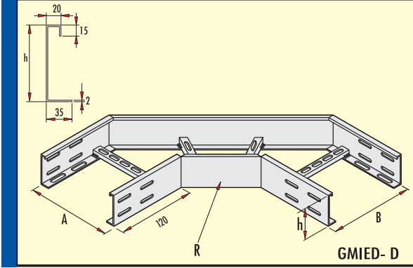
90° Dönüş Elemanı 300 Radius (h=100 mm) 90° Flat Bend Element Radius 300 (h=100 mm) 90° Квартир Сгибает Элемент
