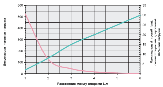
Лоток лестничного типа SL 100x200 S = 1,2 мм
