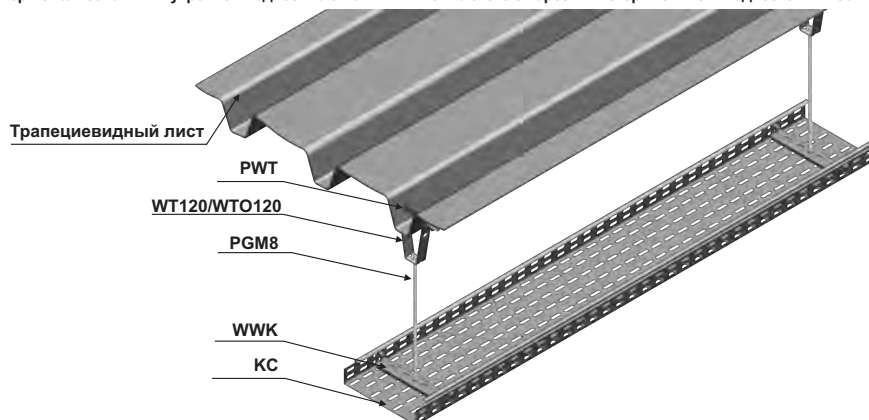
Пример использования внутренней подвески лотка WWK в комплексе с нарезным стержнем PG и подвеской WT 80
