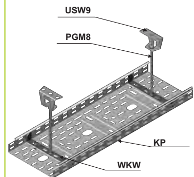
Пример использования внутренней подвески лотка WKW
