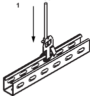
Пример крепления при помощи цепи и подвески WBC40 к швеллеру CWC40H47.
